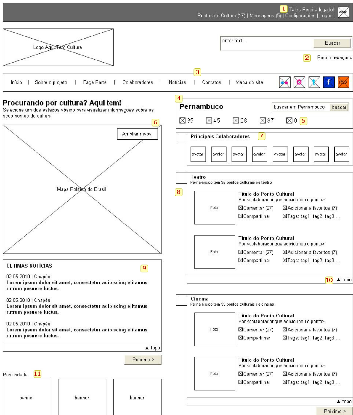
Fig. 02 - Wireframes
